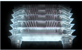
インバータの両面冷却構造
