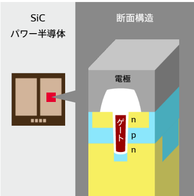
独自の3次元構造(特許技術)
