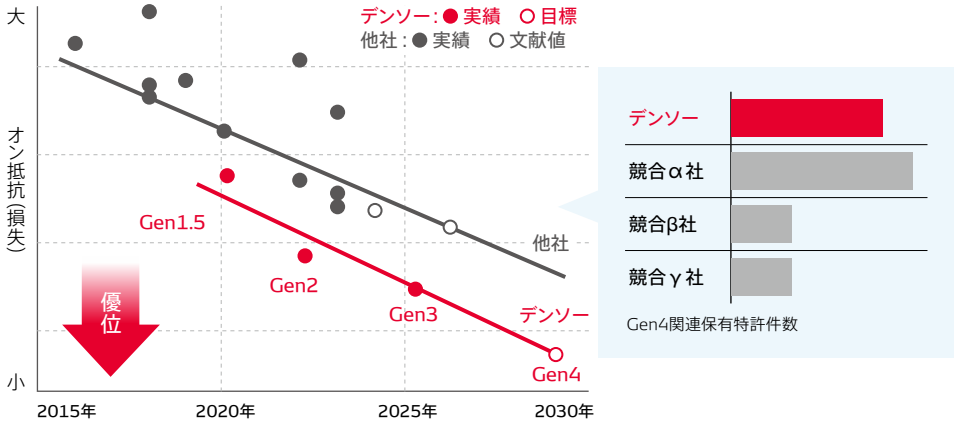
低損失化によるSiCパワー半導体の高性能化
